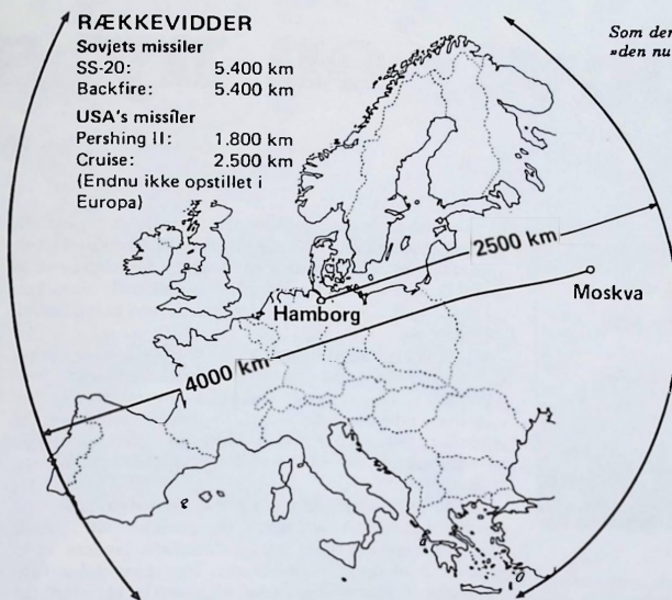
Figur 18: De moderne sovjetiske eurostrategiske våbensystemer, SS-20 og Backfire, kan fra baser dybt inde i Sovjetunionen nå mål overalt i NATO-Europa. NATO har ikke for nærværende modstykke til disse våben og må derfor forlade sig på den amerikanske strategiske afskrækkelse. Den nuværende mangel på balance kunne således synes at indbyde til sovjetiske afprøvningsforsøg. NATO's beslutning om at modernisere sine langtrækkende taktisk-nukleare våben i Europa sideløbende med fornyede rustningskontrolinitiativer skal ses som et skridt henimod tilvejebringelse af balance på dette væsentlige punkt
